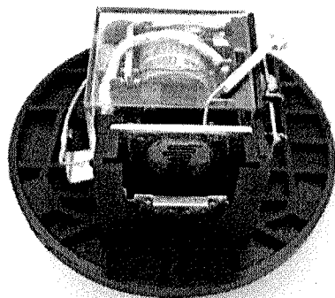
FOTOCONTROLADOR MAGNÉTICO IMAGEM INTERNA
